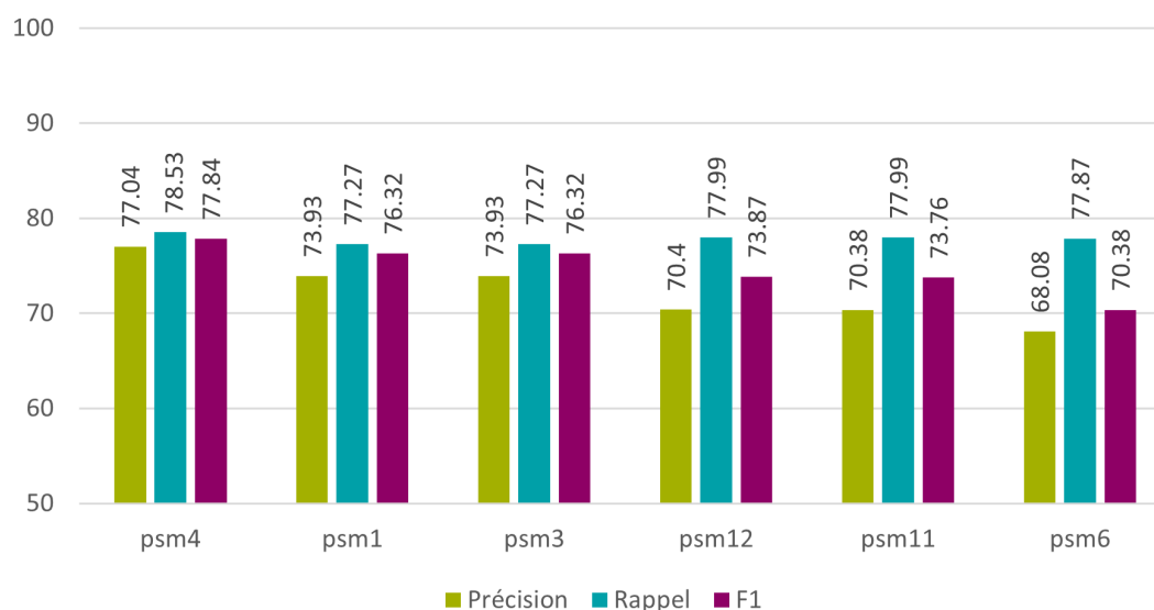
Figure 9 : Tesseract – phase 2 – psm – caractères
