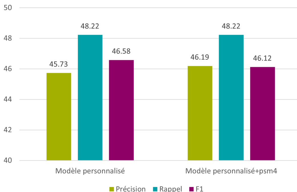
Figure 25 : Tesseract – modèle personnalisé – caractères
