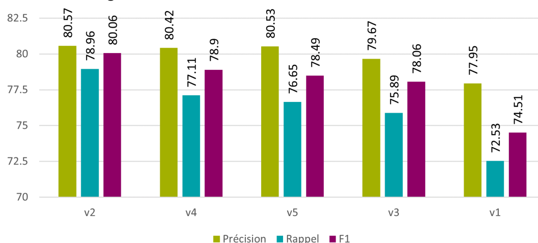
Figure 18 : Tesseract – correction brute – caractères
