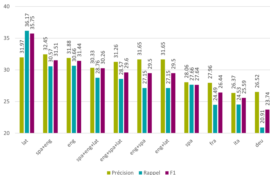
Figure 7 : Tesseract – phase 2 – modèles de langues – mots
