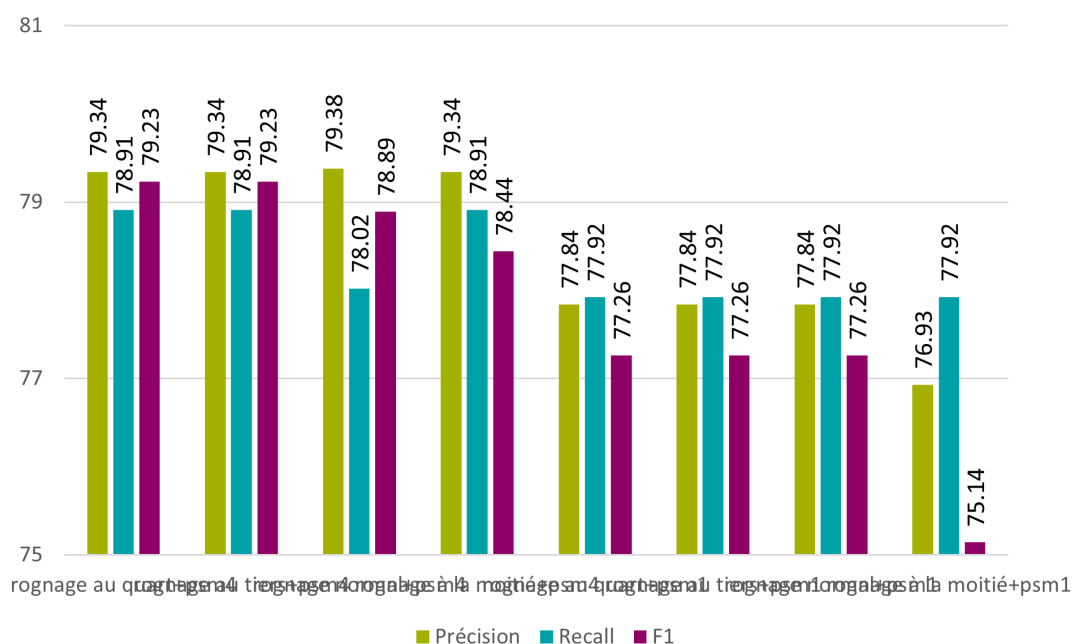
Figure 16 : Tesseract – pré-traitement intelligent – caractères
