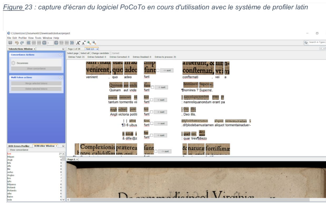
Figure 23 : capture d'écran du logiciel PoCoTo en cours d'utilisation avec le système de profiler latin
